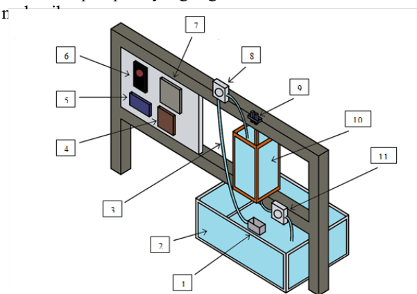
Gambar 4. Perancangan Mekanik .
